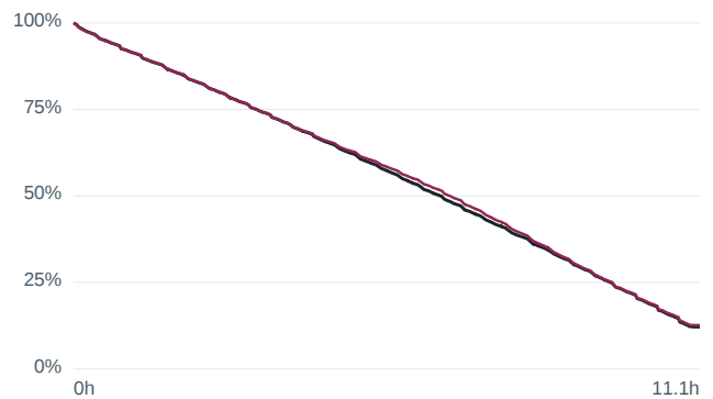
m448 UDDS at 10 °C
