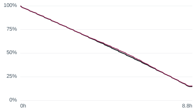
m80 UDDS at 0 °C
